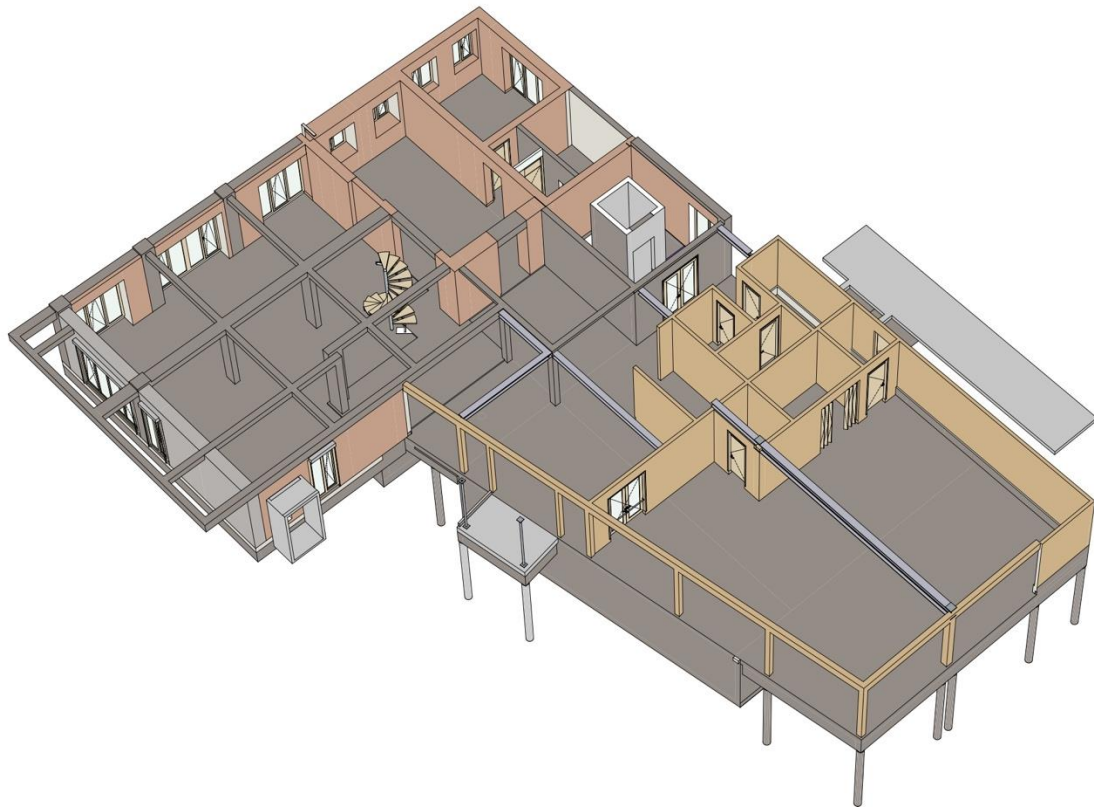
ERDGESCHOSS
